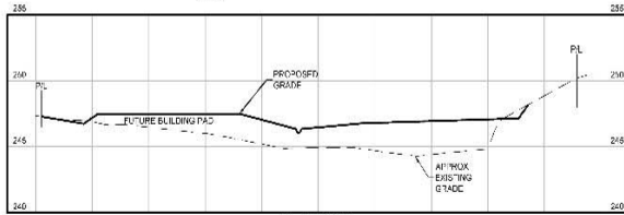
C-PROFILE SCALE: H: 1"=20' V: 1"=5'
