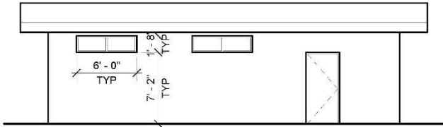
Elevation 1
