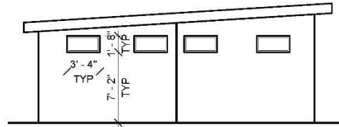
Elevation 4
